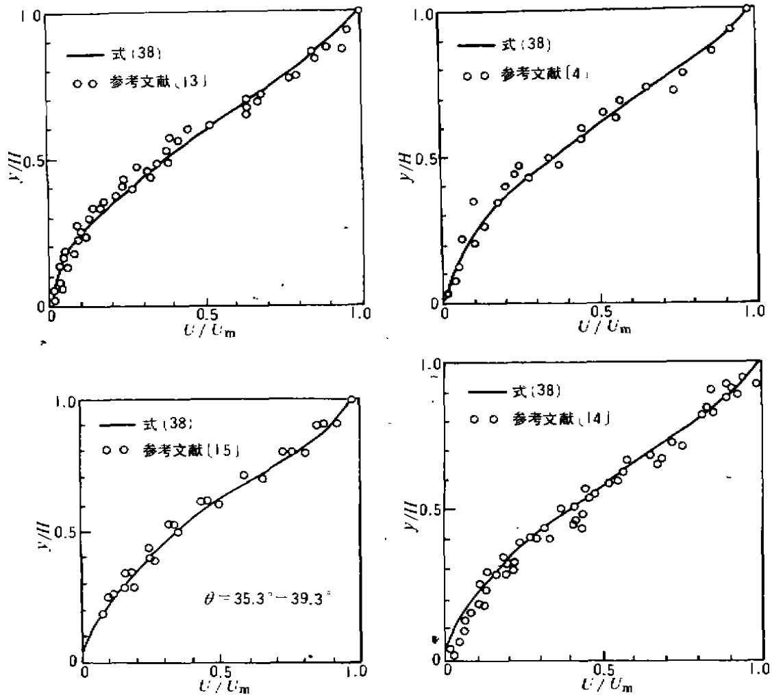
图2 流速分布计算与实测的比较
