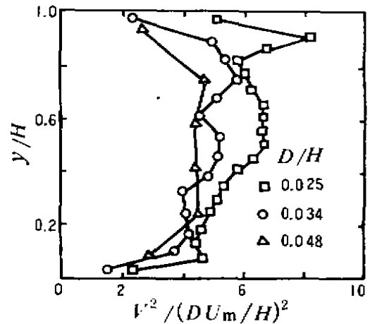
图1 无粘颗粒流脉动速度均方值的分布
