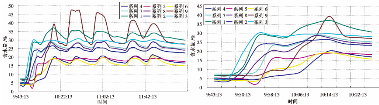
图7 不同时间和部位土体含水量变化曲线(图例系列数与图1中的探头编号一致)
