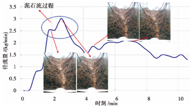
图2 第一个 10 min 泥石流形成图 Fig. 2 Process of debris flow in the first 10 min
