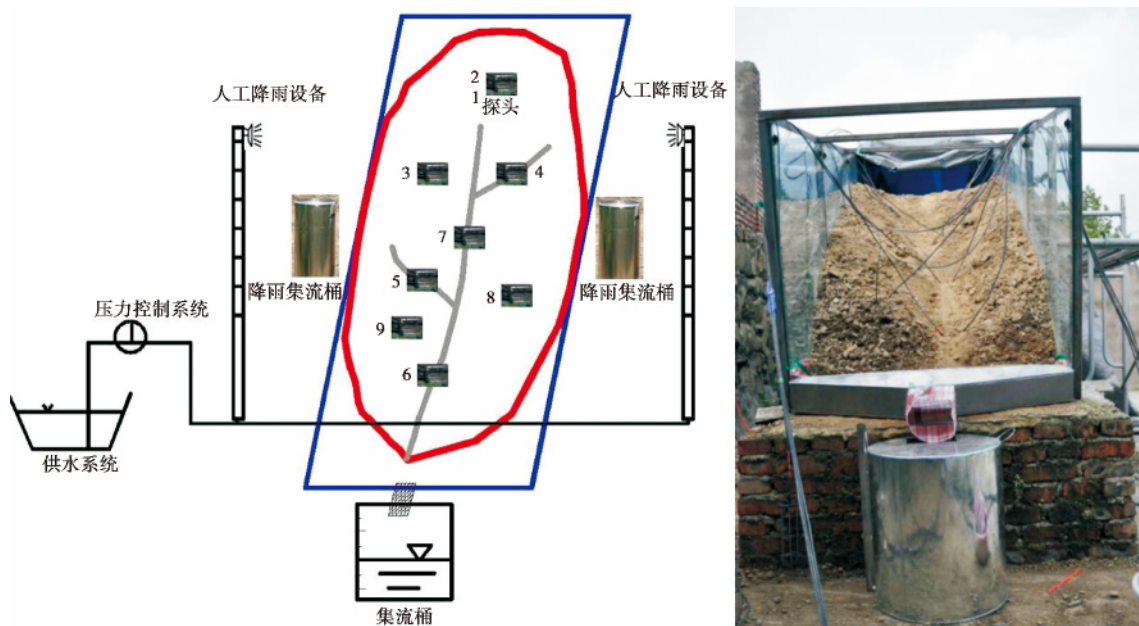
图 1 传感器埋设位置与试验装置
