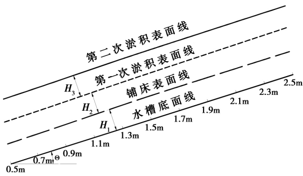
(注: 图中 H_1 表示沟床厚度 H_2 表示单次淤积时相对沟床淤积厚度 H_3 表示连续淤积时第 2 次相对第 1 次淤积厚度; H_1 、 H_2 、 H_3 分别为水槽横剖面左、中、右三个测量位置处的厚度平均值)
