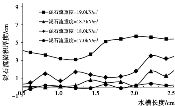
图 6 不同泥石流重度条件下淤积厚度对比图
