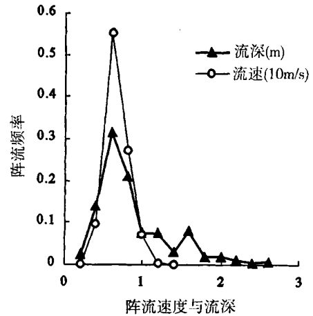
图3 真实阵流的速度与流深
