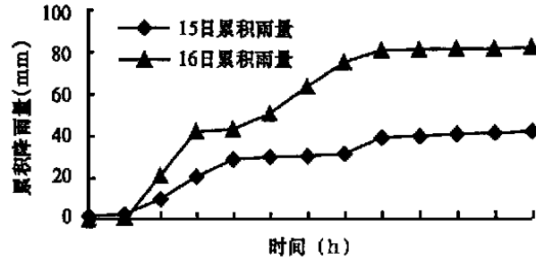
图2 1994—06—15~16, 0~12时的累积雨量过程
