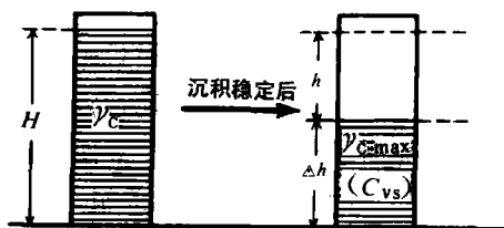
图2 泥石流流体沉积过程示意
