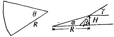
图 3 锥体要素
